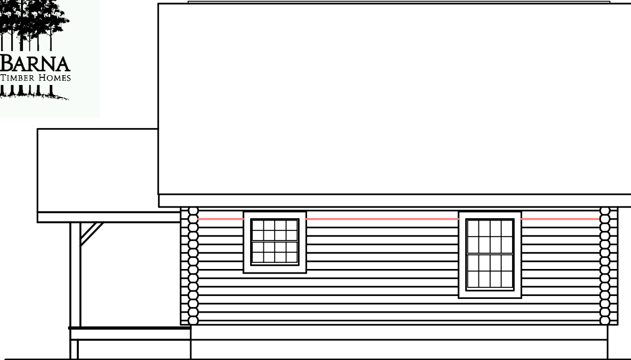
RIGHT ELEVATION
