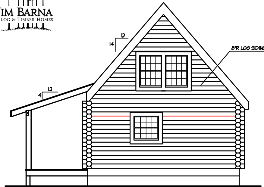
RIGHT ELEVATION
