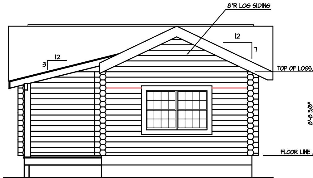
RIGHT ELEVATION
