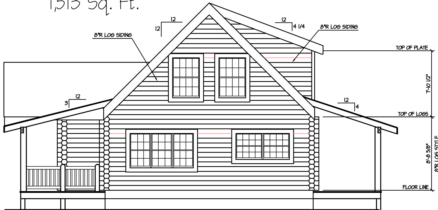
RIGHT ELEVATION
